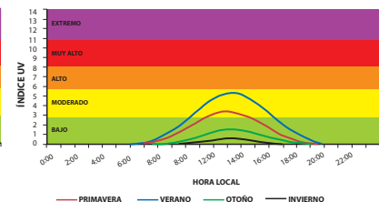
RADIACIÓN ULTRAVIOLETA COMPORTAMIENTO DIARIO ESTACIONAL ESTACIÓN PUNTA ARENAS
