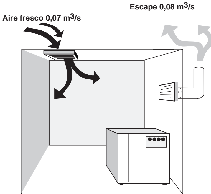
Figura 5.5: Ventilación para máquina abierta
