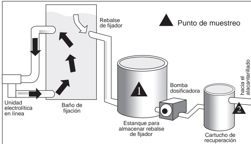
Figura 4.2: Configuración de sistema para recuperación en línea de plata (incluyendo como sistema de control un cartucho de recuperación) (The Silver Council, 1997a; 1997b; 1997c)
