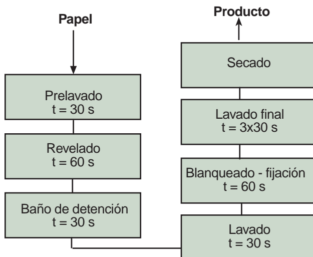
Figura 2.2. Esquema de proceso de impresión a partir de negativos en color
