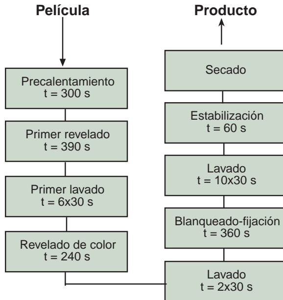
Figura 2.5. Secuencia de etapas de proceso de revelado de transparencia (tres etapas)
