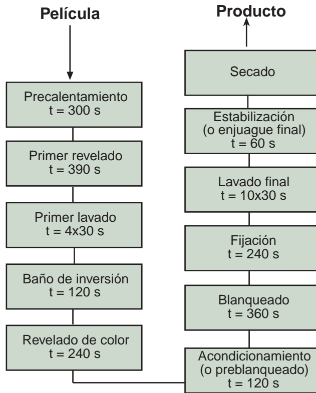
Figura 2.4. Secuencia de etapas de proceso de revelado de transparencias (seis etapas)
