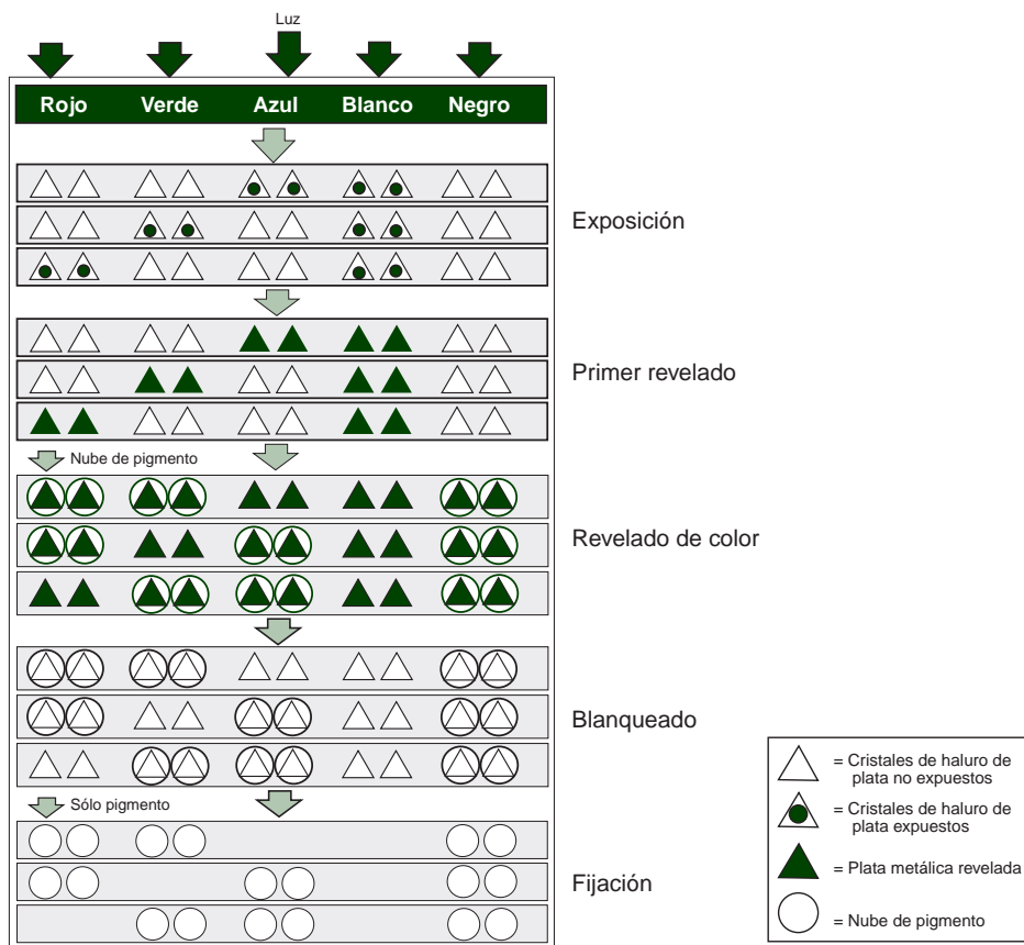
Figura 2.3. Formación de imagen de color durante el procesamiento (Kodak, 1997)
