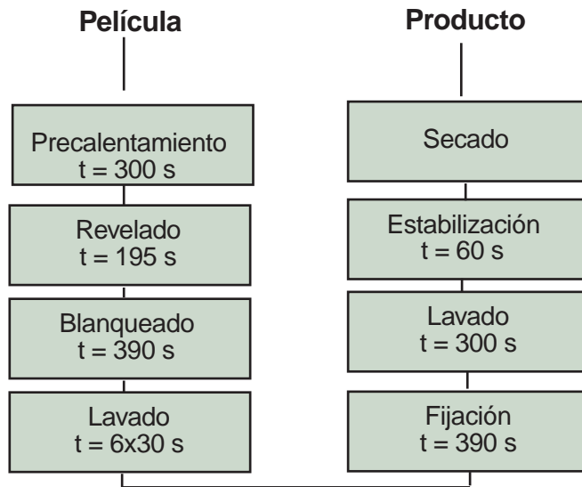
Figura 2.1. Secuencia de etapas de proceso de revelado de negativos de color (USEPA, 1991; JOBO Fototechnic, Inc., 1997)
