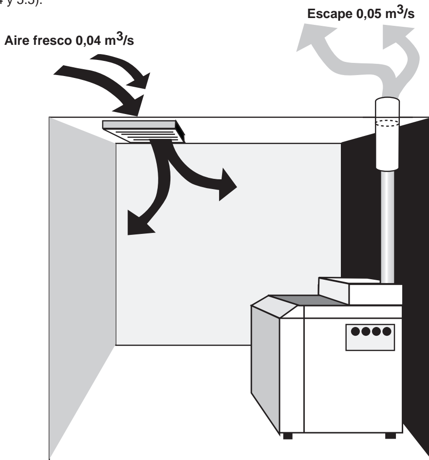
Figura 5.4. Ventilación para máquina cerrada
